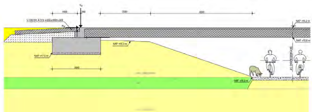
Figuur 6.3.13.A Variant onderdoorgang N525, fundering op staal
