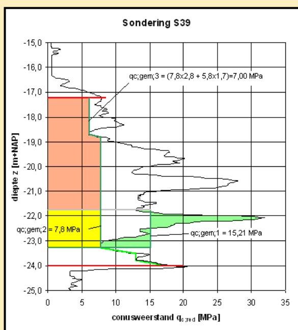
Figuur 7.3.16 Berekening paalpuntweerstand volgens Koppejan
