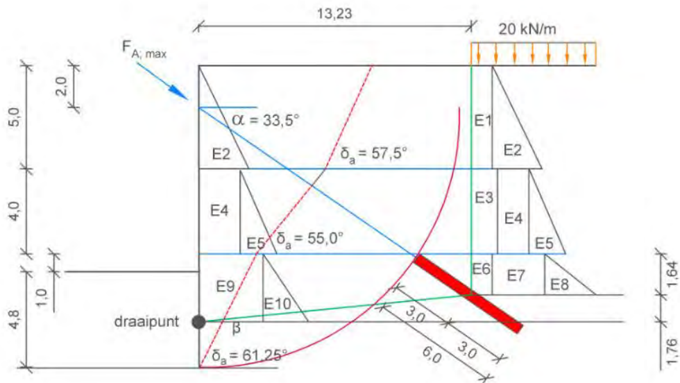
Figuur 8.8.8 Ontwerp positie grout-tanker
