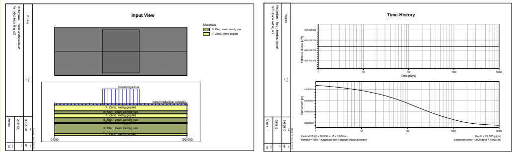
Figuur 7.3.19 Berekening zakking paalgroep met MSettle
