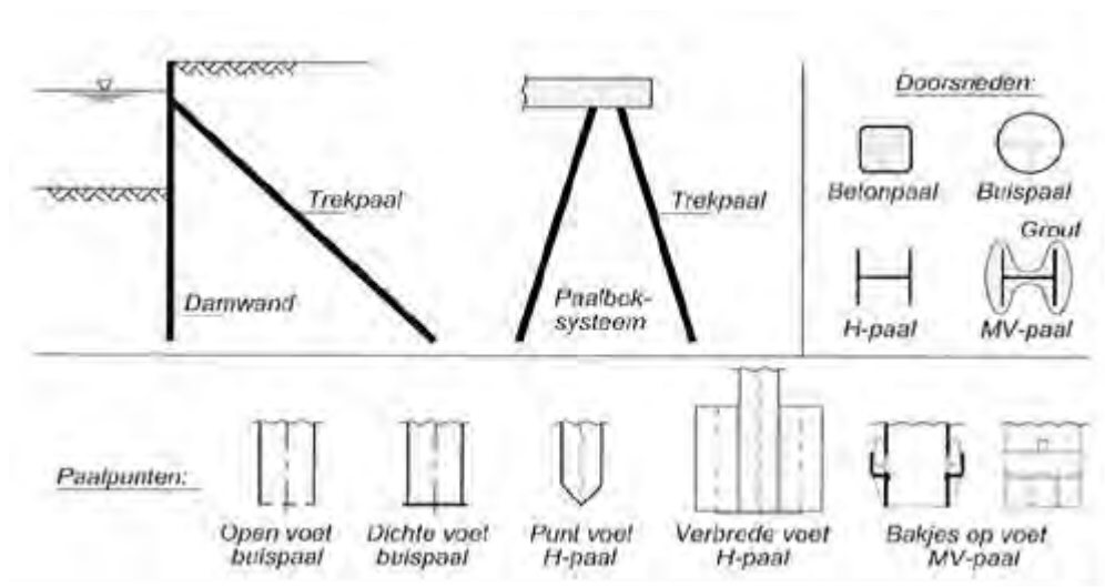
Figuur 10.3.6 Trekpalen (bron: Handboek Kademuren [10.1])
