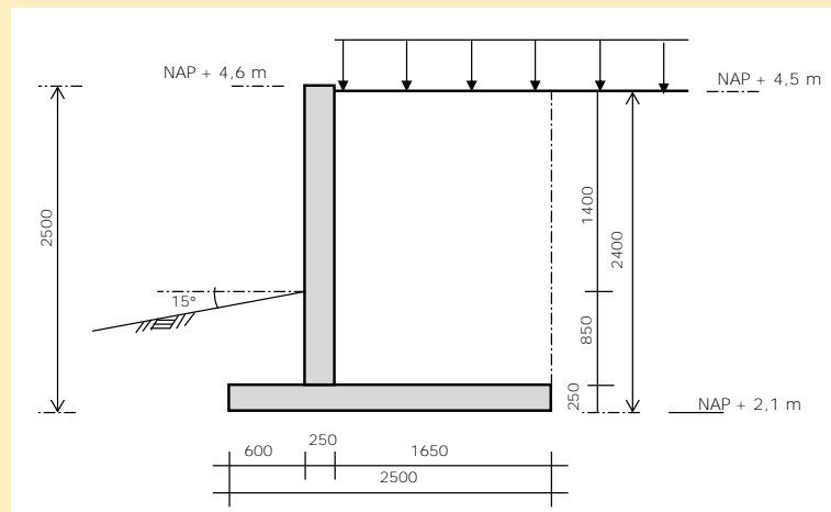
Figuur 6.6.5. Schematisering Variant L-muur ver- breiding A2
