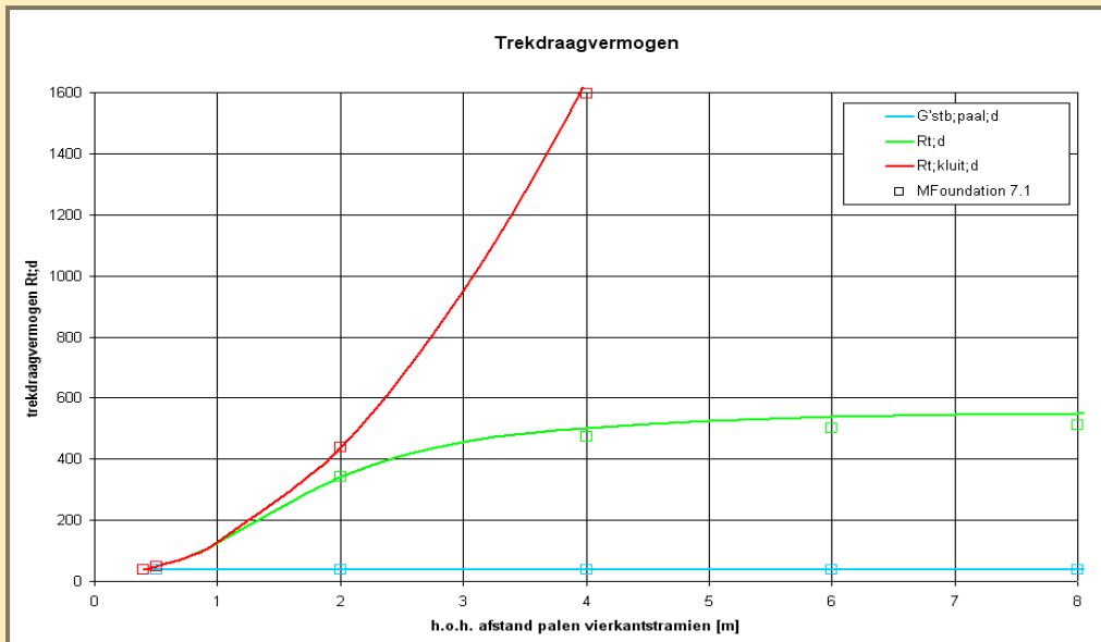
Figuur 7.4.11 Invloed h.o.h. afstand palen op trekdraagvermogen
