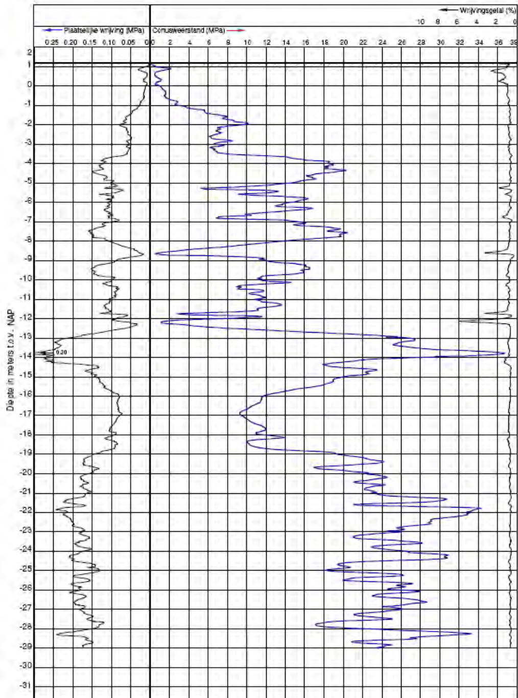
Figuur 8.A.11 Sondring 23
