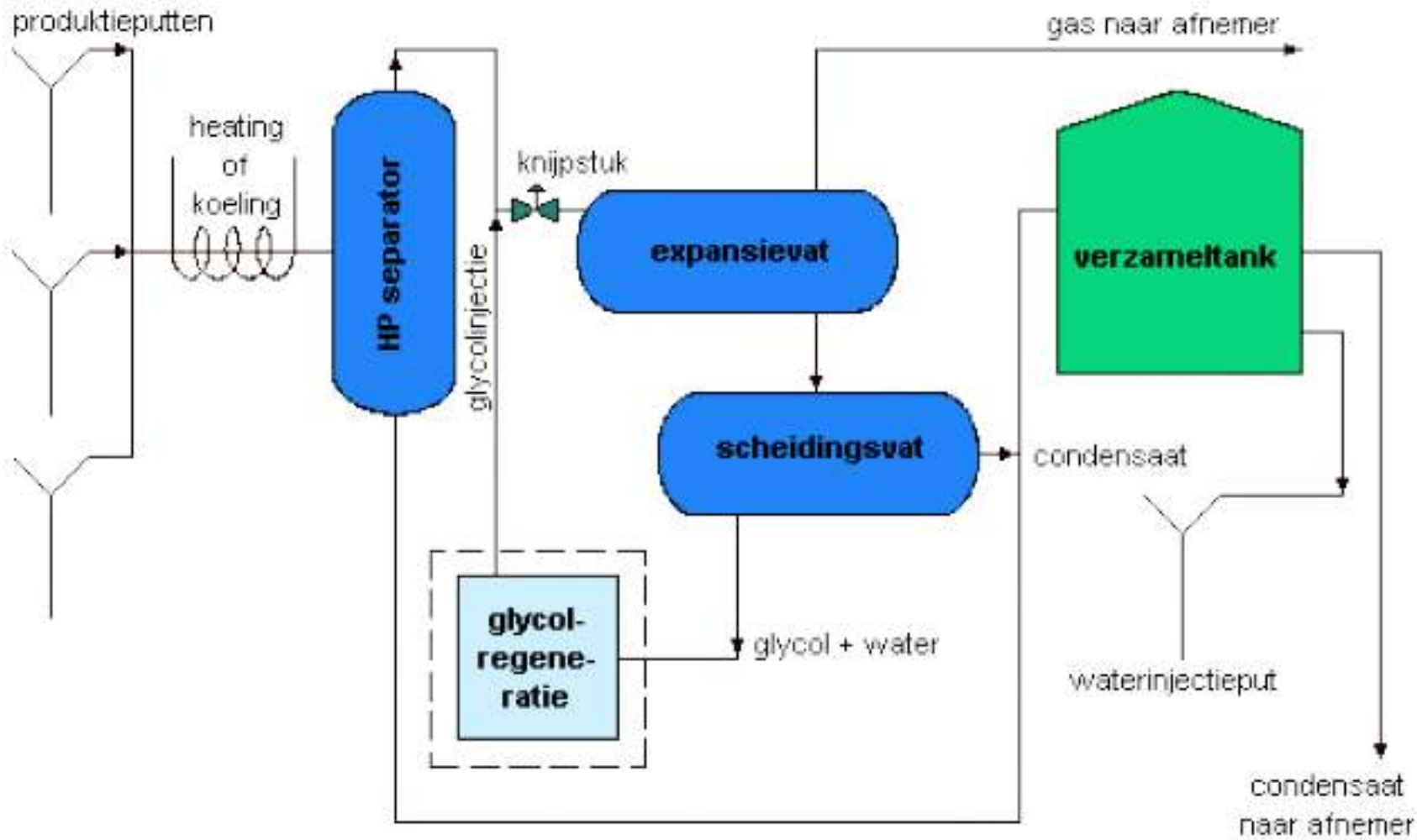
Principeschema gasbehandelingsinstallatie - expansie en glycolinjectie
