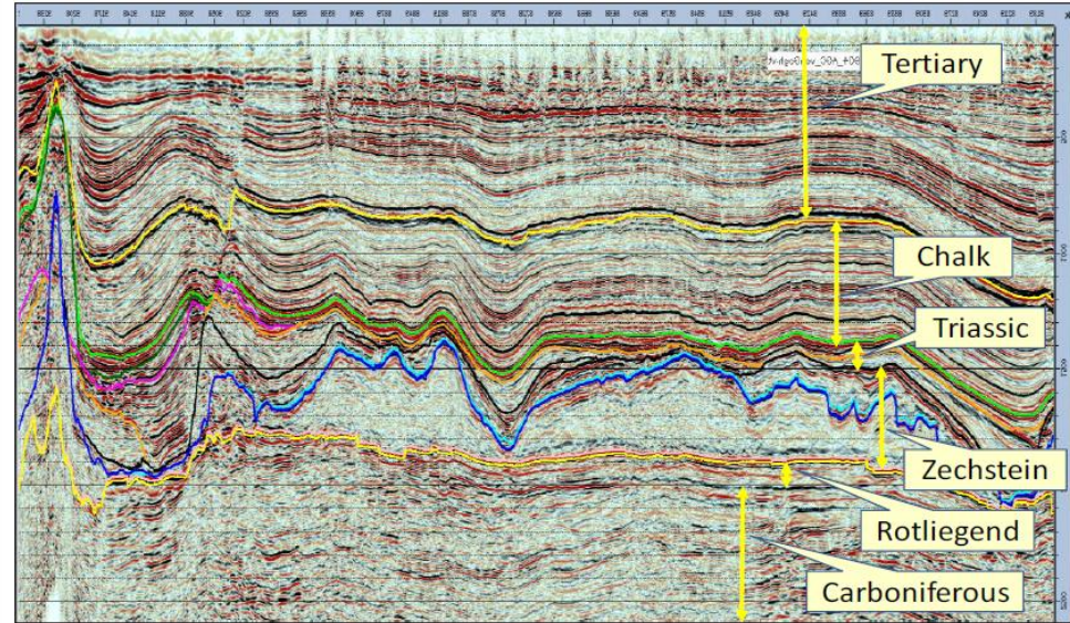
Veld doorsnede
