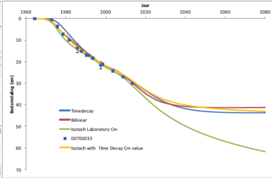
Compactie Modellen
