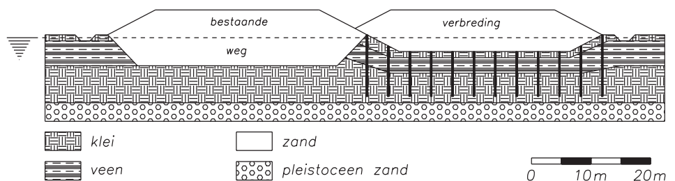
Figuur 1.1 Principe zandophoging op maaiveld met verticale kunststofdrains
