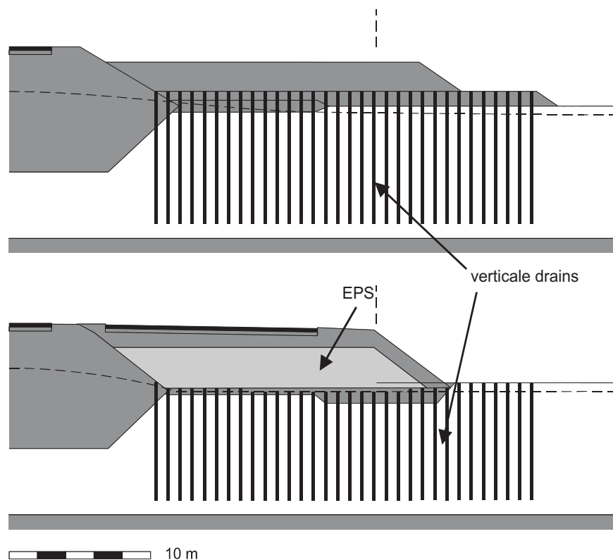
Figuur 4.1a: Schematische wijze van uitvoering
