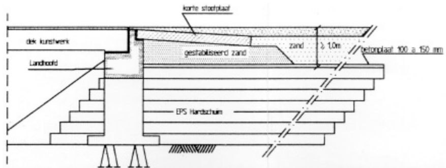
Figuur 4.1b: Voorbeeld EPS ophoging met zandbed en belastingspreidende betonplaat bij een overgangconstructie naar een viaduct (uit [14])
